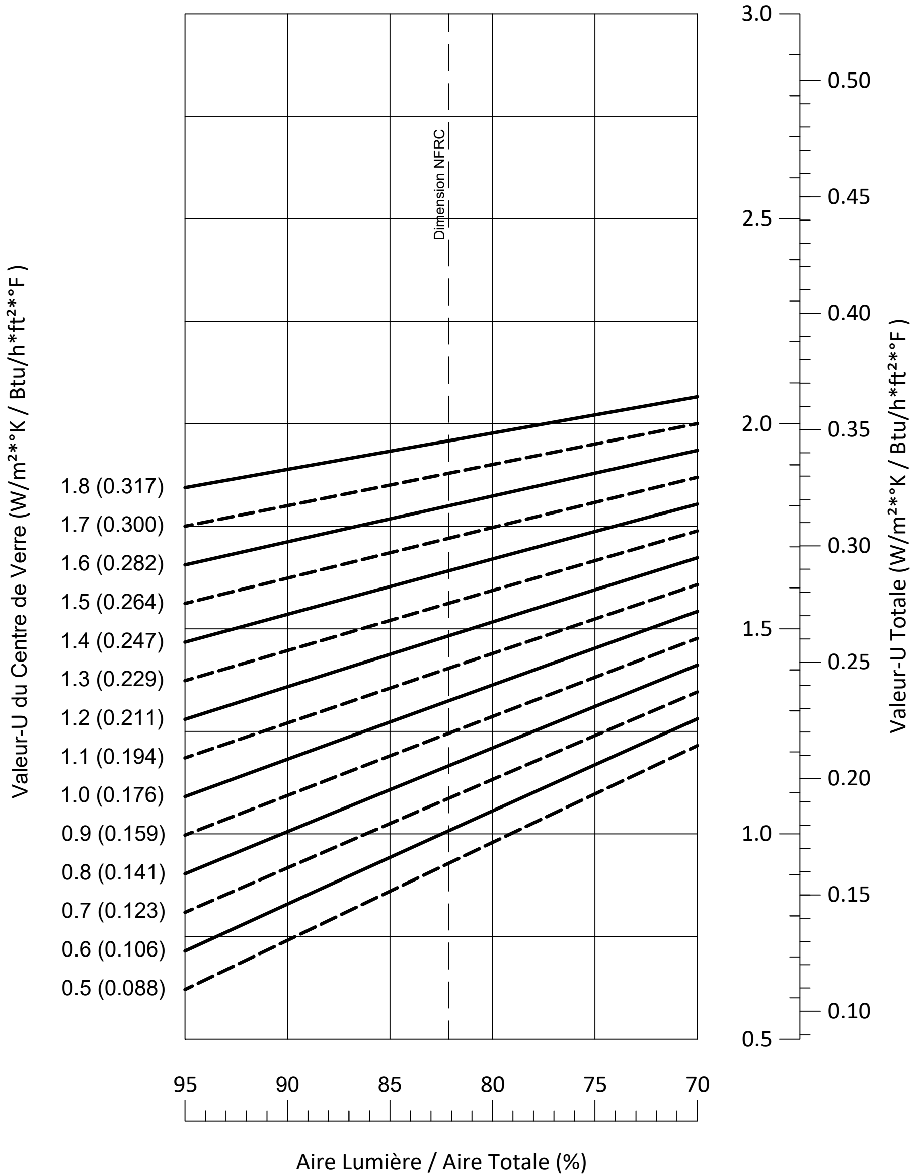
Valeur-U Totale contre Pourcentage de l'Aire Lumière
